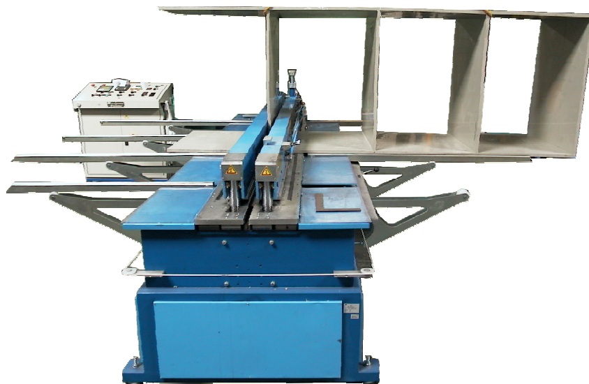
Soldadura automatica vertical
