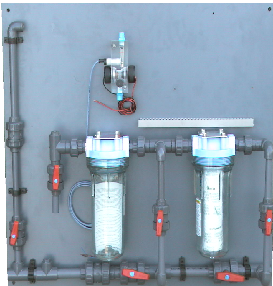
Cuadro dosificador
